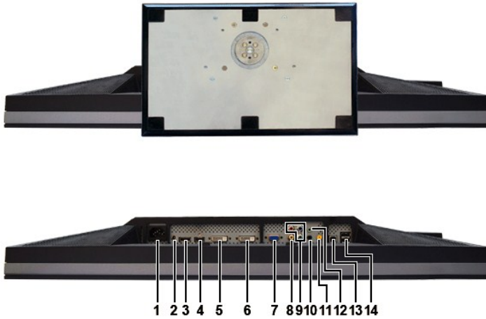
底視圖
